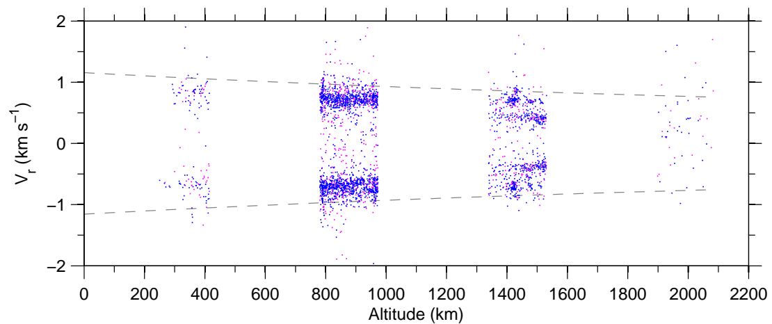
Figure 7: Doppler-velocity v altitude , 02 Apr–08 Apr 2007.
